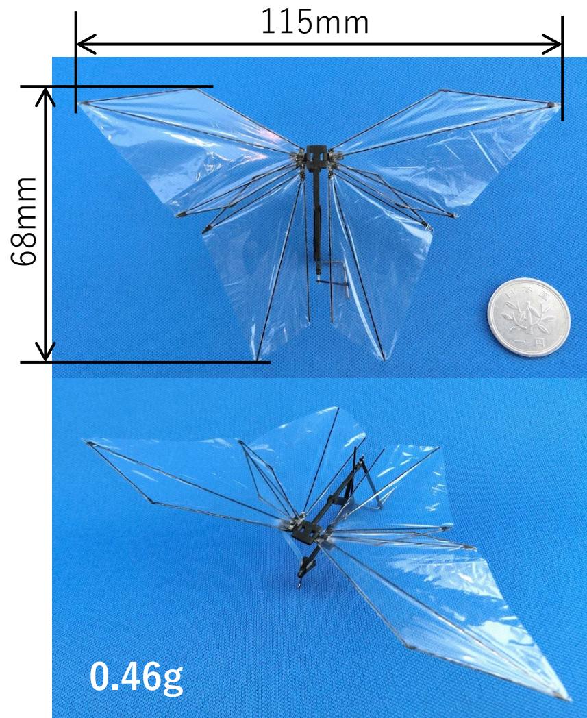
テイクオフ・モデル（ゴム動力）
