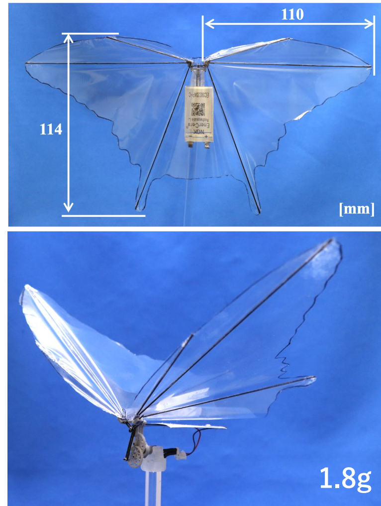
フリーフライト・モデル（モータ, バッテリ搭載）
